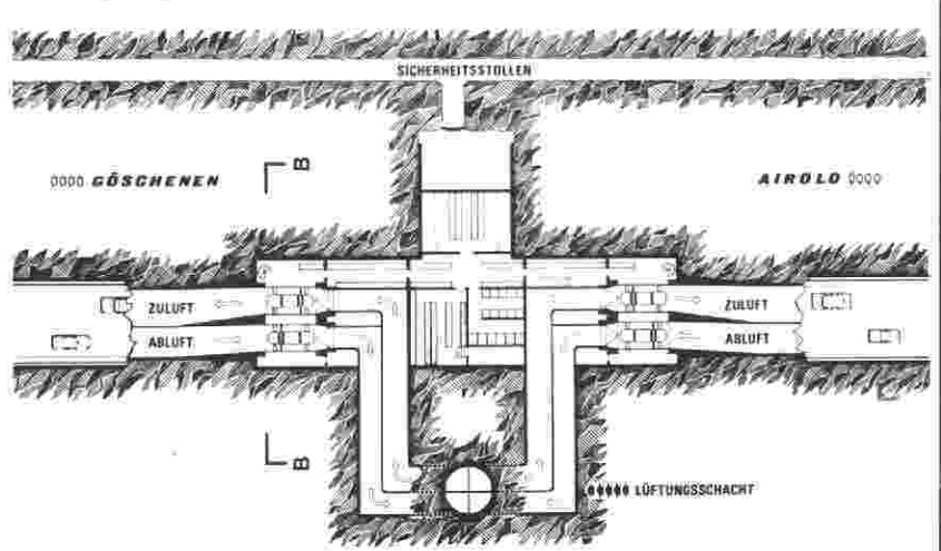
GRUNDRISS VENTILATIONSZENTRALE
