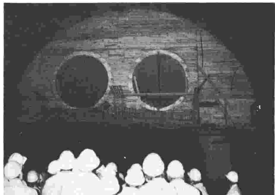
Die über 3 Meter Durchmesser aufweisenden Luftkanäle in der Ventilationszentrale
