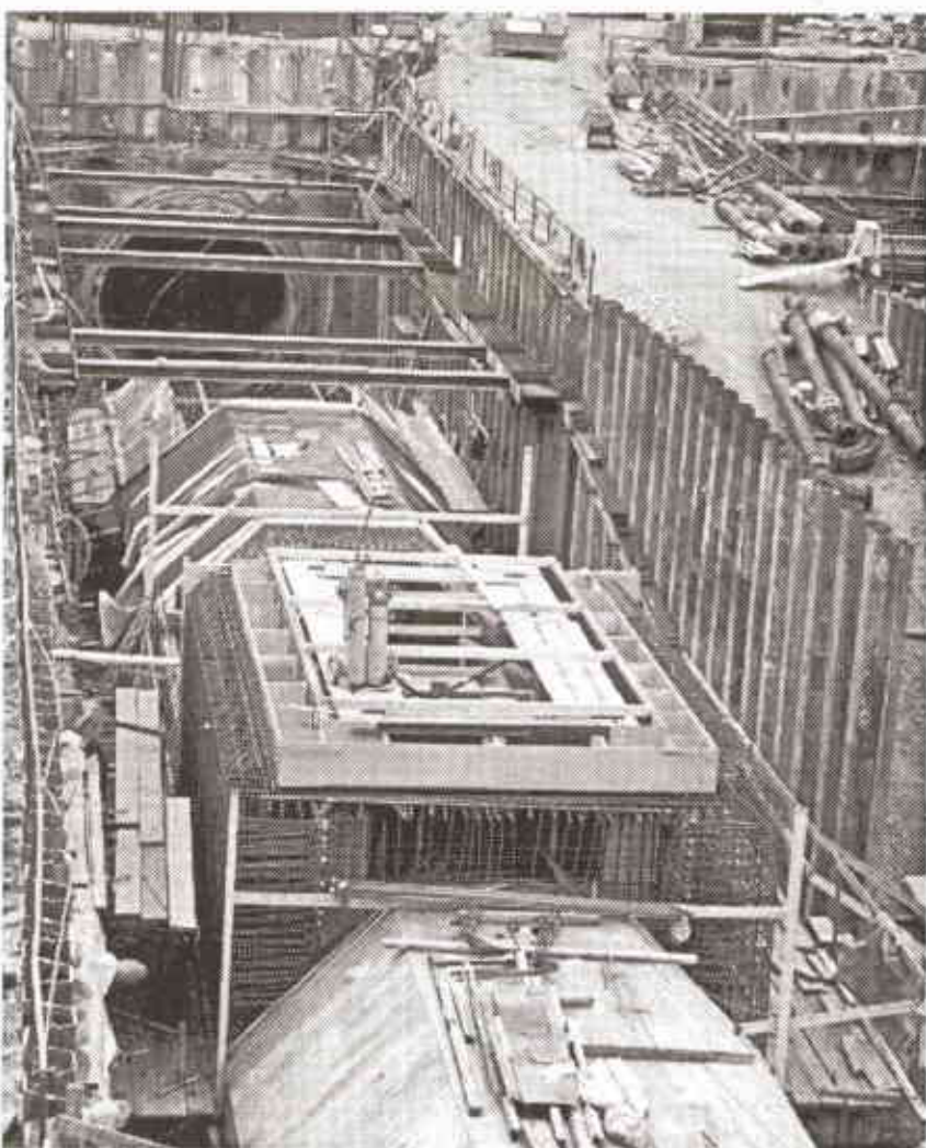
Tunnelröhre für das Personentransportsystem
